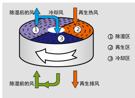
蜂巢工作原理示意图
