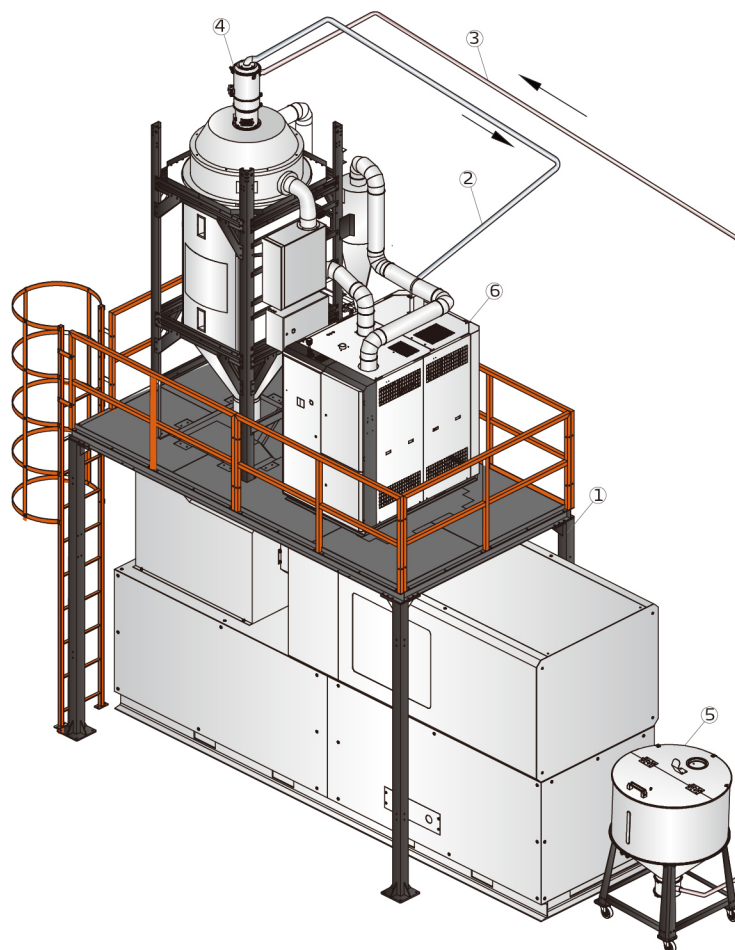
平台送料示意图
