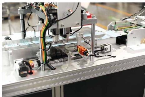
伺服拉耳帶機構
